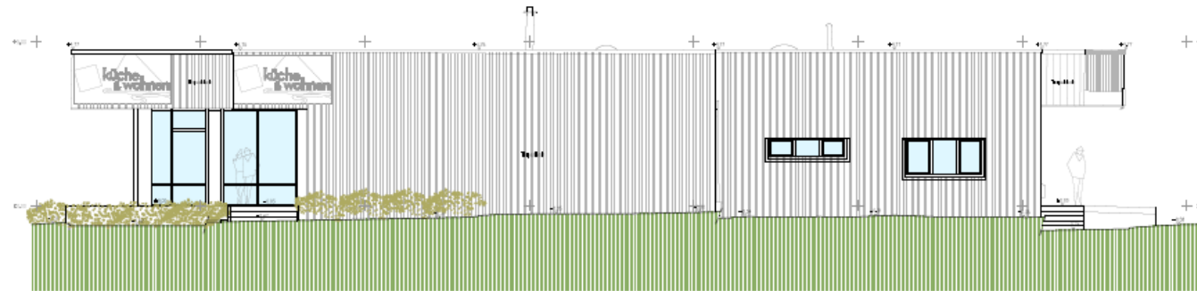
SÜDANSICHT:
