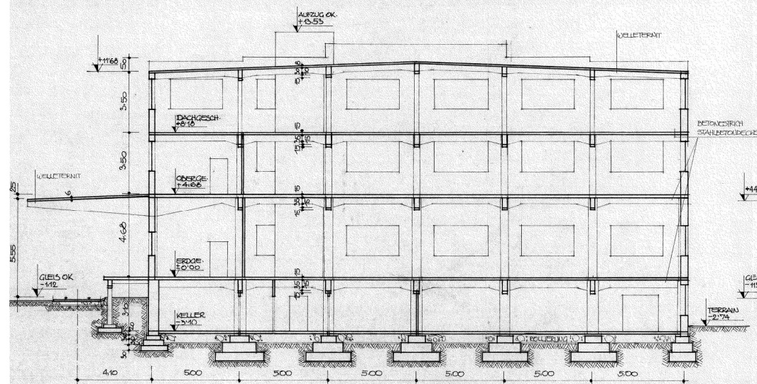
SCHNITT A-A
