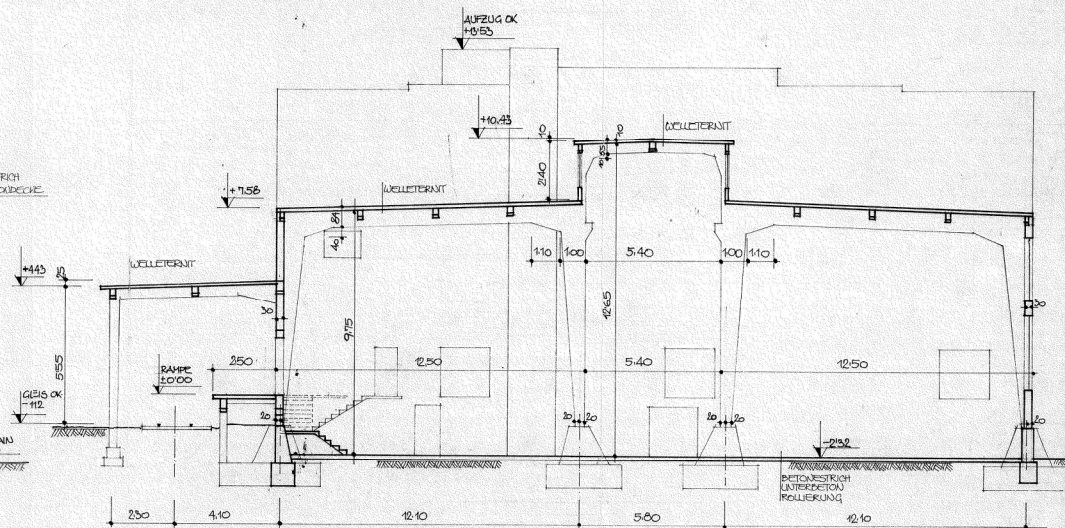
SCHNITT B-B
