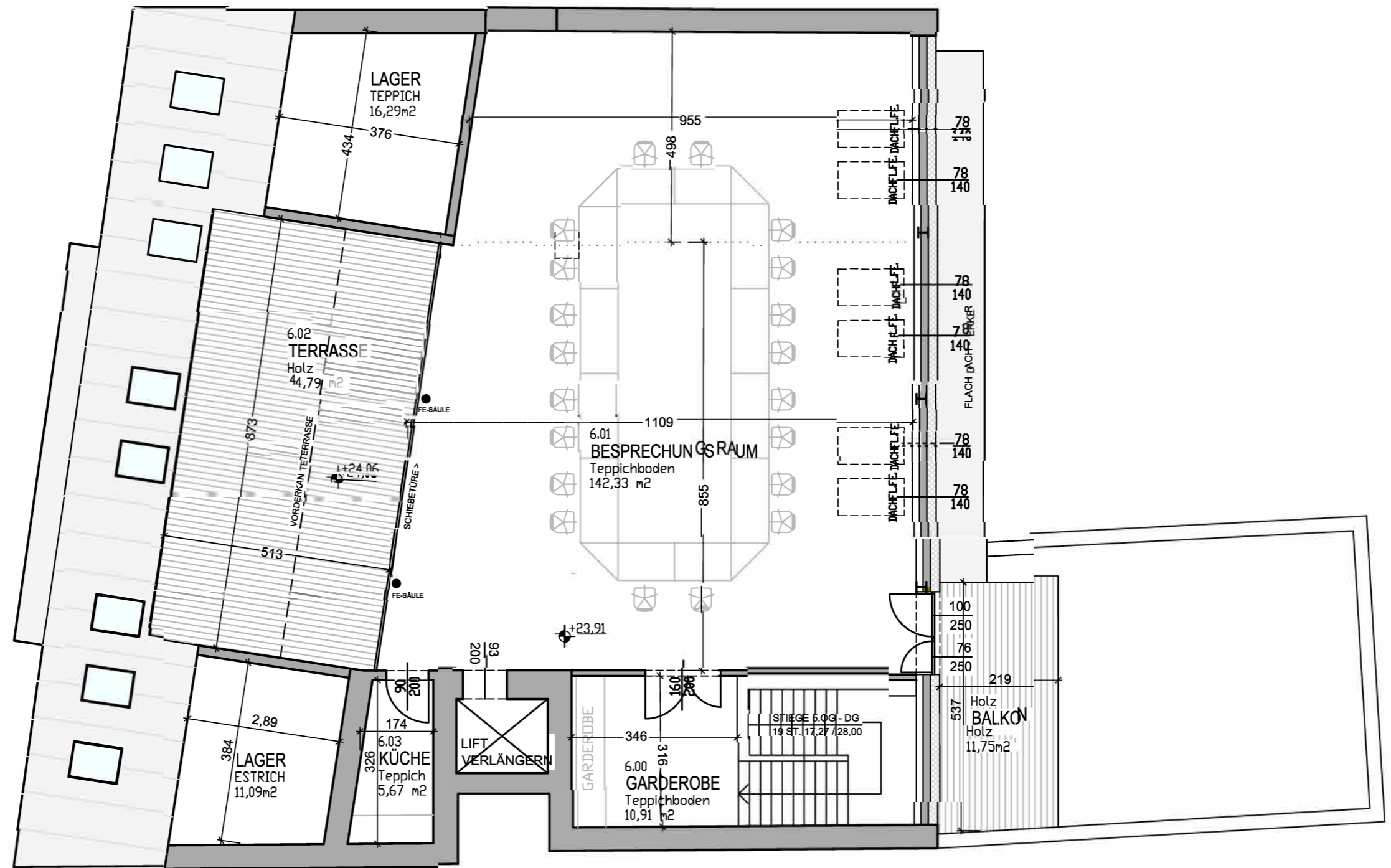
GRUNDRISS DACHGESCHOSS
