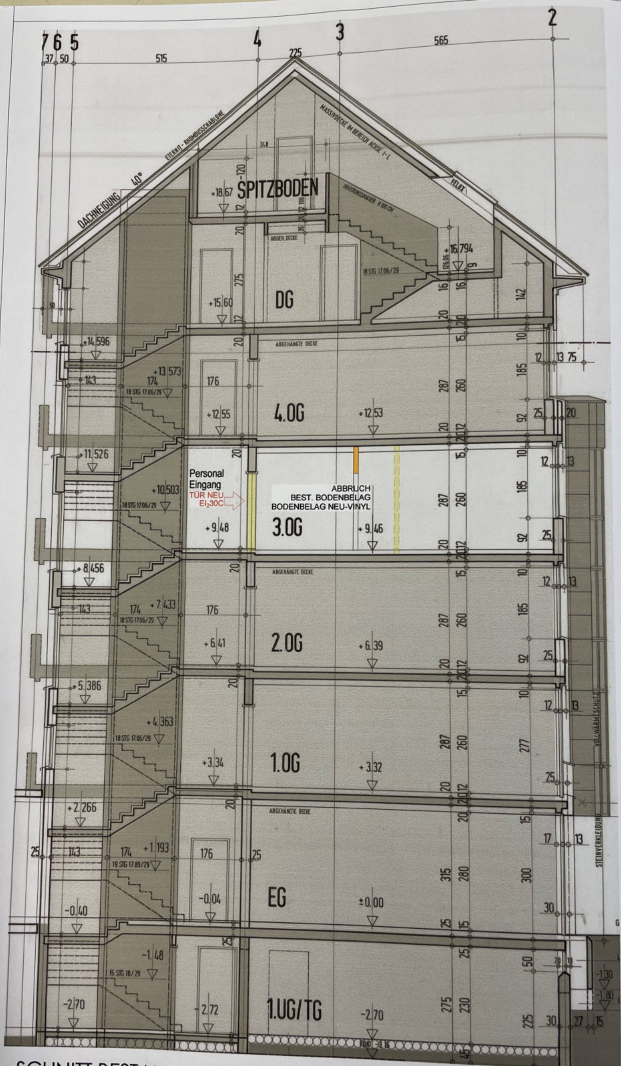
SCHNITT BESTAND
