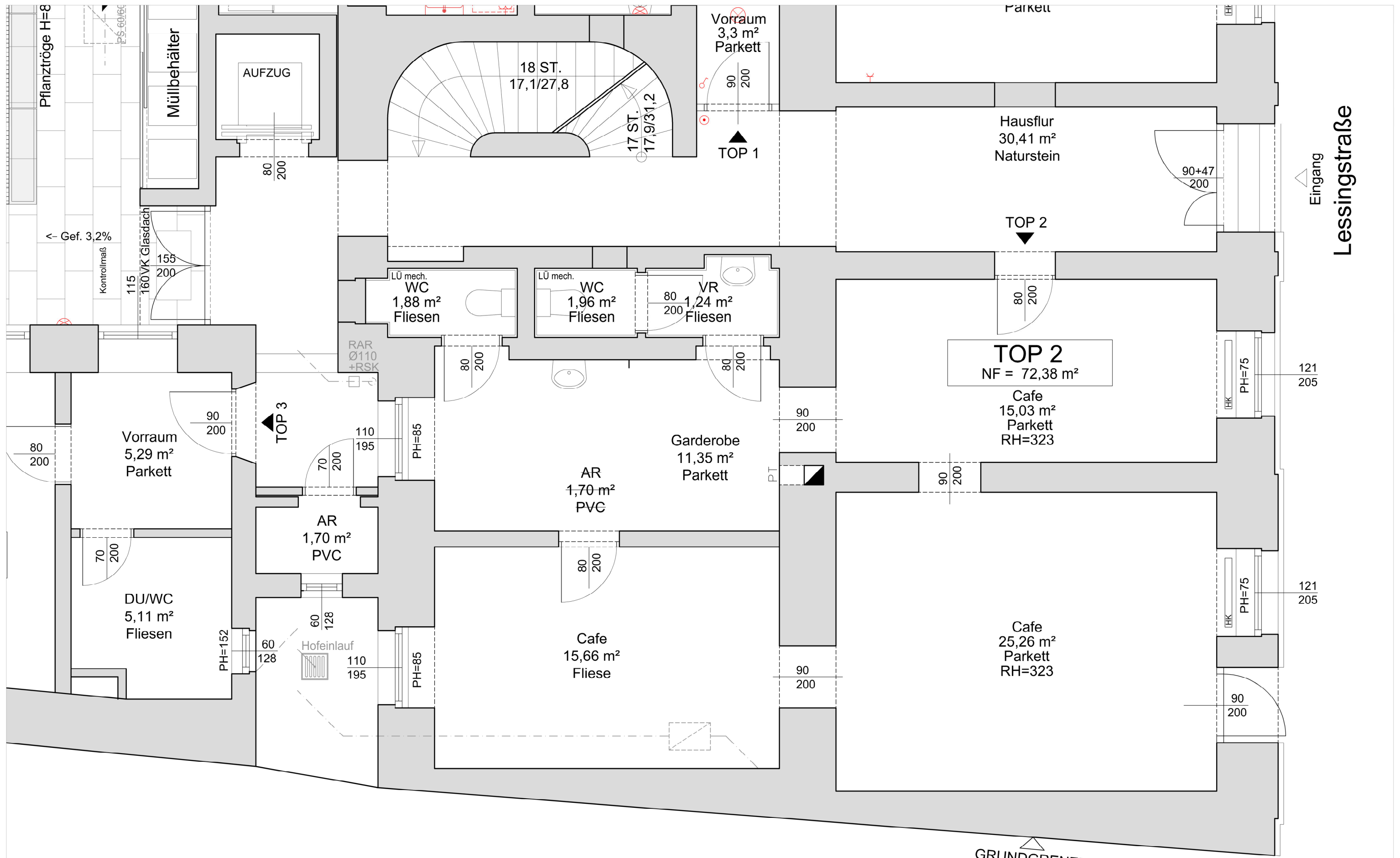
TOP 2 - M 1:50
