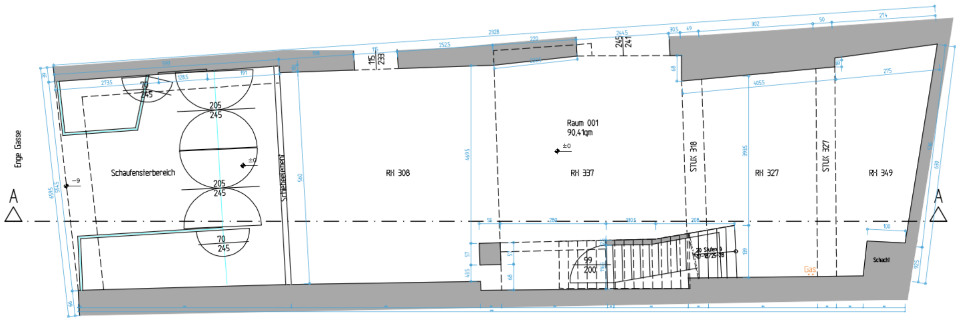
GRUNDRISS EG
